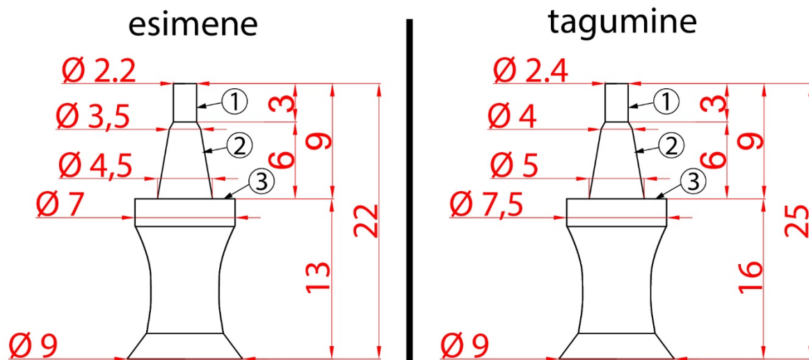
Krossinaela joonis
