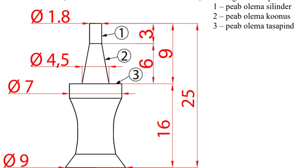
Naela joonis
